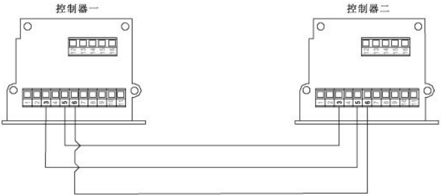
双门互锁连接图
